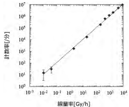
図6 光子計数率の線量率依存性 6)
