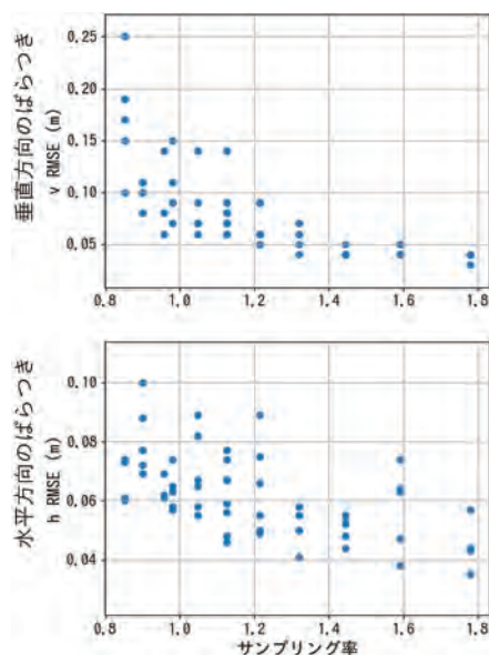
図5 サンプルング率と近似曲線からの点群のばらつき
