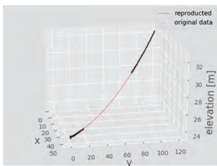
図4 送電線点群およびあてはめたカテナリー曲線点群として再現されていない区間が曲線で補間されている
