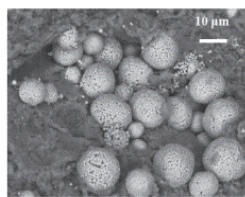
黄鉄鉱の拡大図
