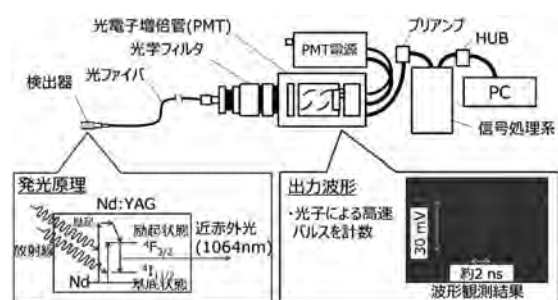
図 3 光子測定装置の構成図
